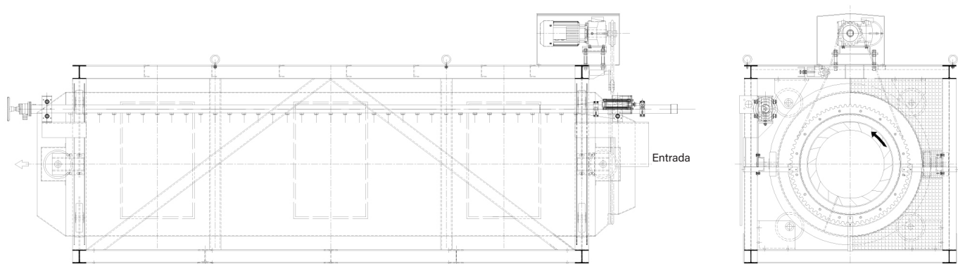
Rotoscreen L: Ideal para lavar los residuos de la despulpadora a través de una puerta directa.
