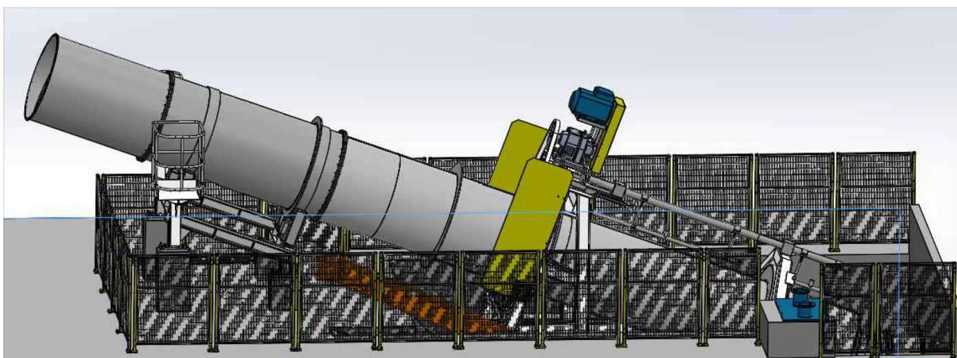
Rotoscreen I: Solución ideal para recibir y tratar los residuos de cualquier máquina.
