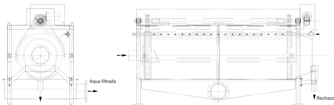
Rotocriba horizontal en posición superior: Para el lavado de los residuos de la purga.
